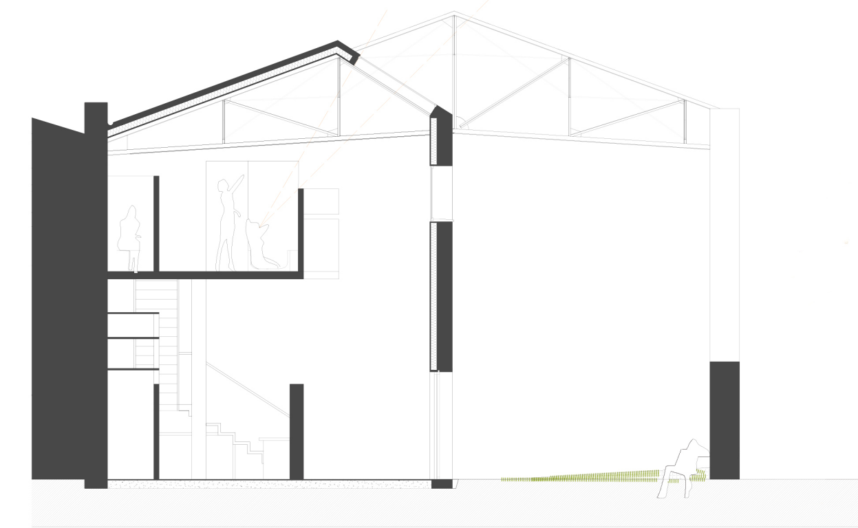
COUPE AA'
