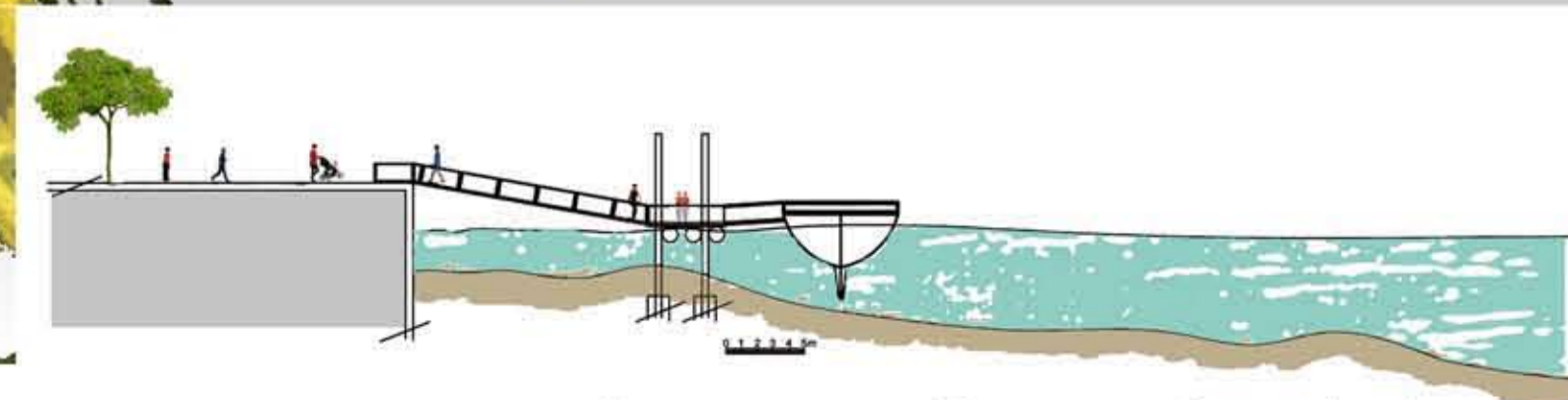
Coupe d'un ponton flottant à marée basse
