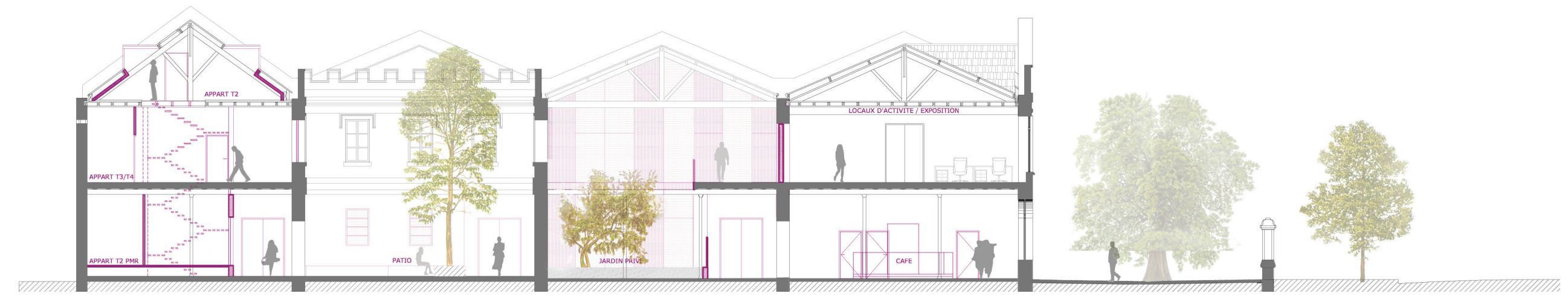
Coupe transversale - I:200
