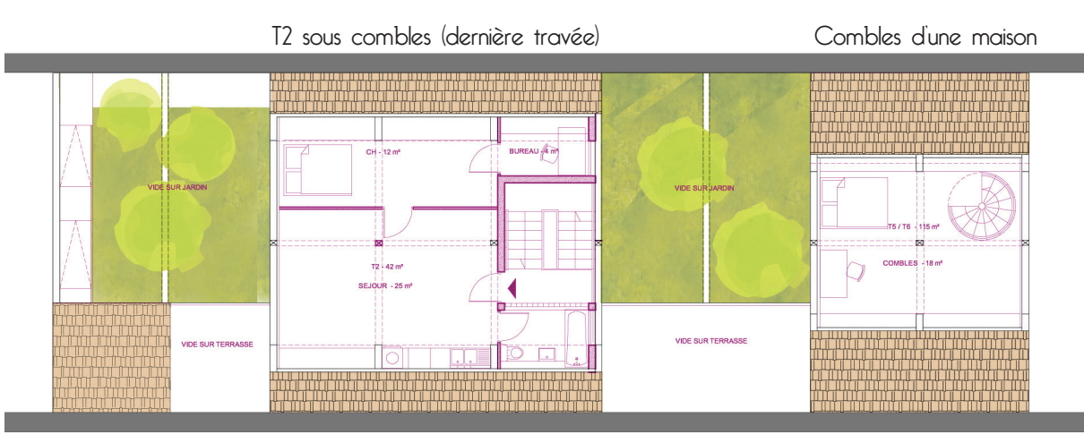
Plan sous combles I:200
